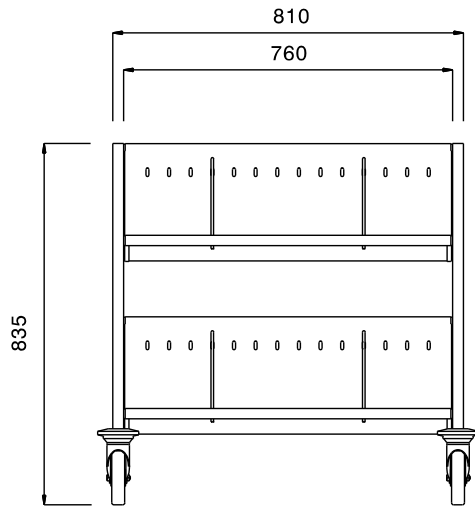
Front aanzicht
